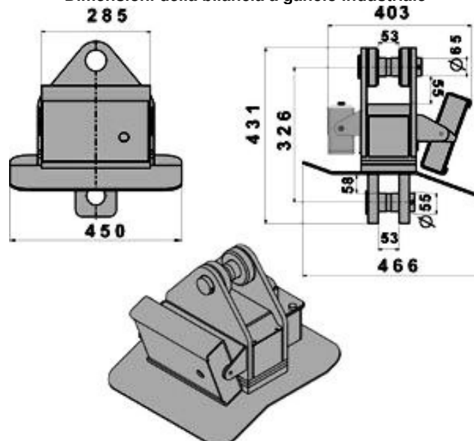
Dimensioni della bilancia a gancio industriale
